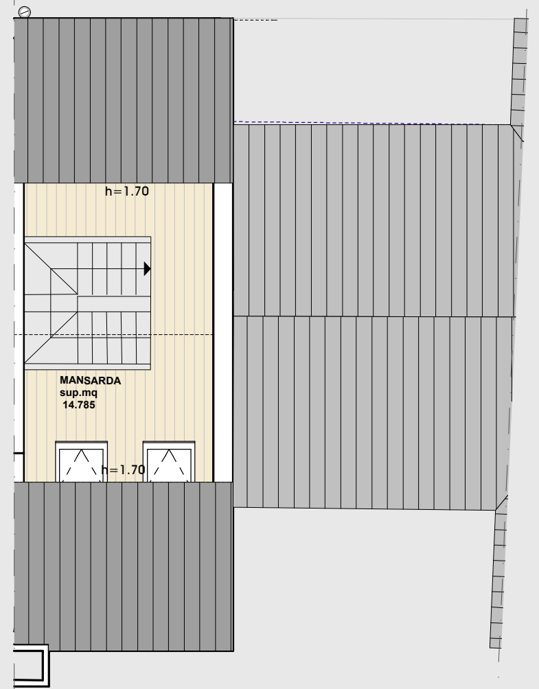
pianta piano sottotetto
