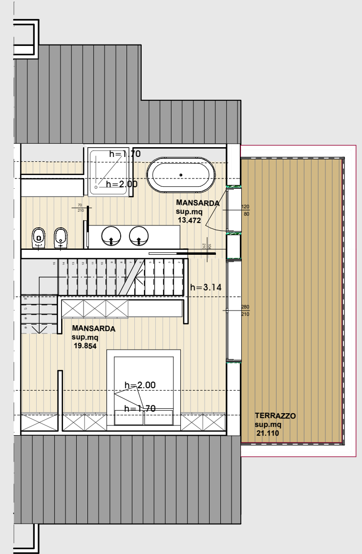
pianta piano sottotetto
